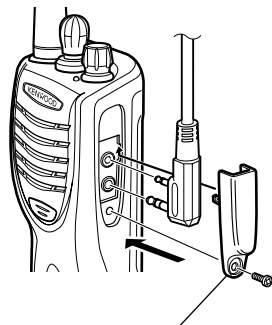
Fixierdeckel für Lautsprecher-/ Mikrofonstecker
