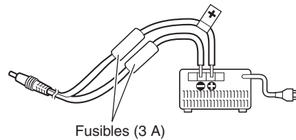
Fusibles (3 A)
