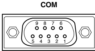
Rückansicht
