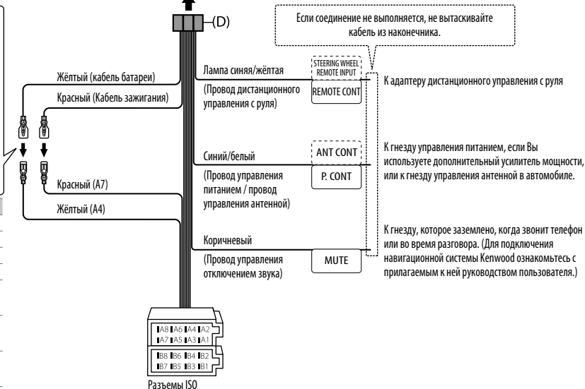
Разъемы ISO
