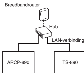
Figuur 4: KNS-systeemconfiguratie in een thuis LAN-omgeving
