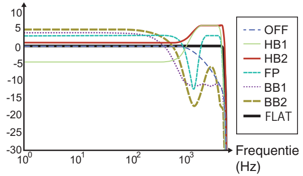
RX-karakteristiekcurve
