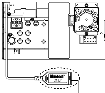
Adaptador Bluetooth (KS-UBT1)
