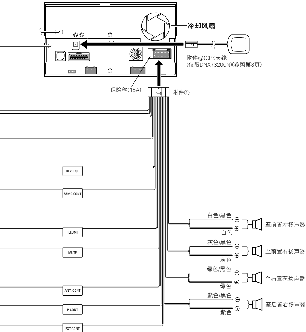
后视图
