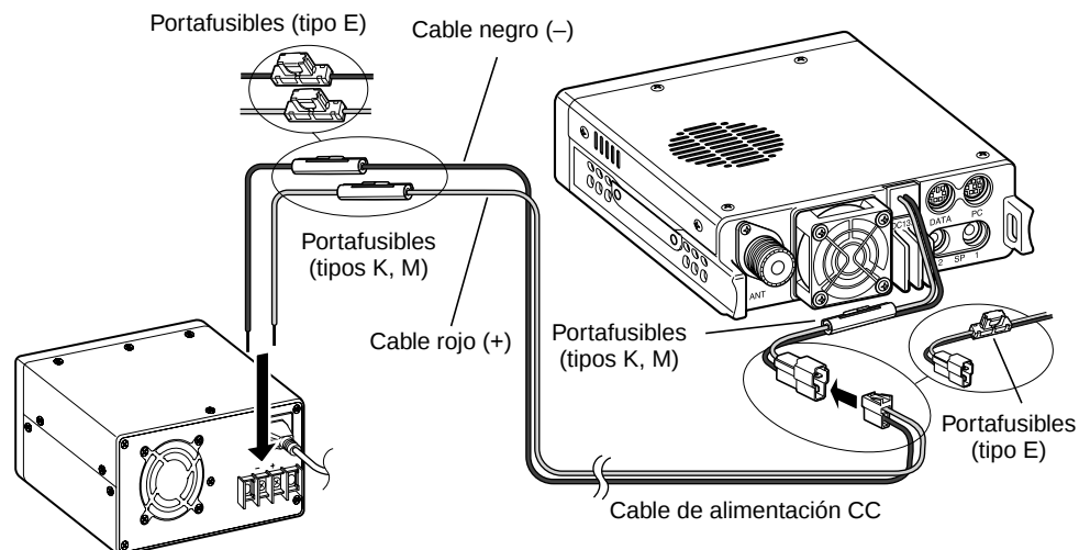
Fuente de alimentación DC regulada
